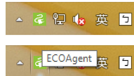
圖2：ECOAgent圖示
