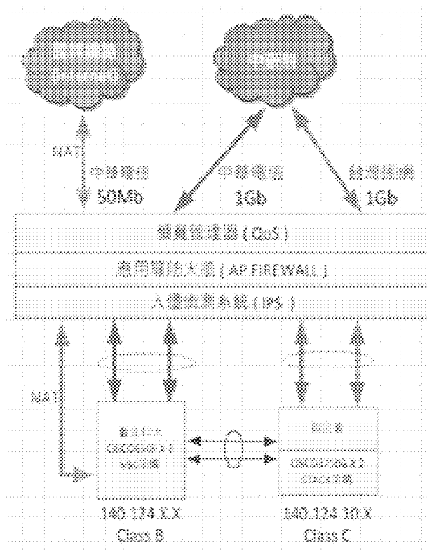
目前聯外網路架構
