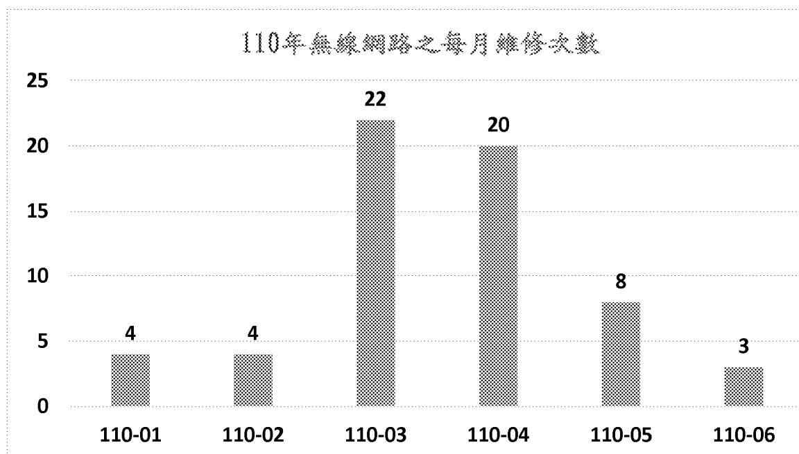
圖八、無線網路 110 年 1 至 6 月報修次數統計圖
